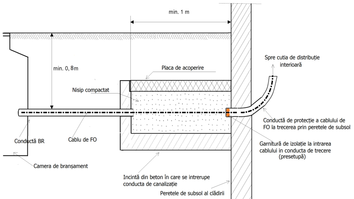
Fig. 5 Introducerea cablului în clădire folosind „întreruperea/disipare de gaz”
