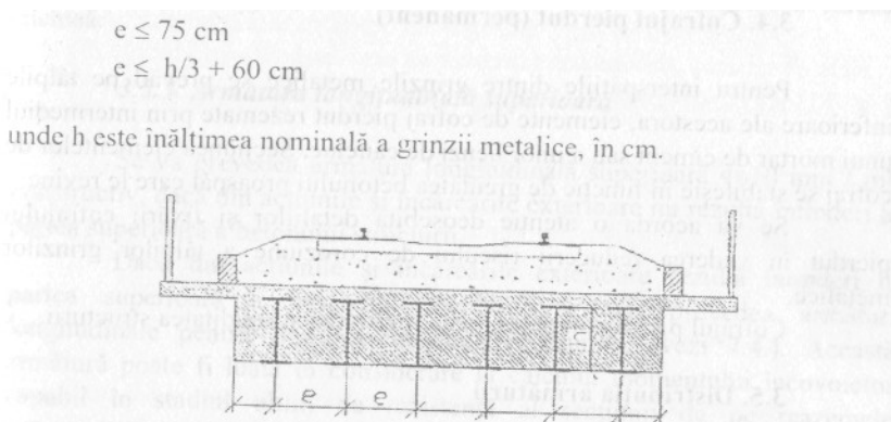
FIGURA 1: Schema secțiunii transversale pentru un tablier cu grinzi metalice înglobate în beton
