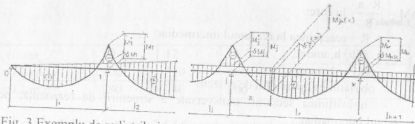
Fig. 3 Exemplu de redistribuire a momentelor încovoietoare pentru structură continuă cu 3 deschideri inegale
