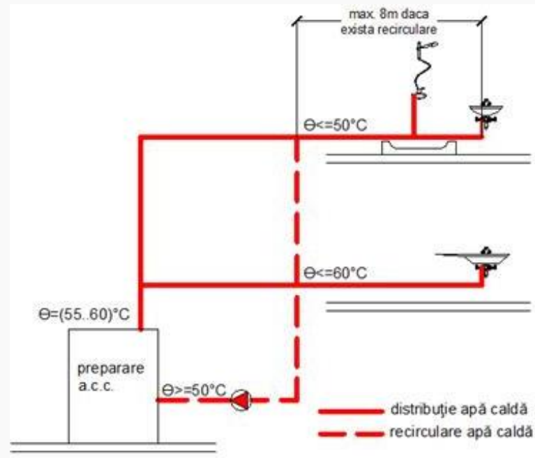
Figura 11.2 Preparare individuală a apei calde, fără recirculare, temperatura maximă la punctele de utilizare
