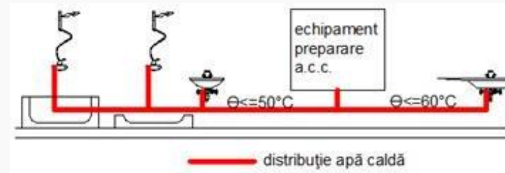
Figura 11.3. Preparare individuală a apei calde, cu recirculare (traseul de distribuție este mai lung de 30 m), temperatura apei calde se va menține la minim 50^\circ\text{C} .
