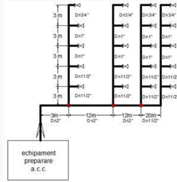
Figura A4.2. Schema de calcul, prezentată de principiu, pentru dimensionarea conductei de recirculare.
